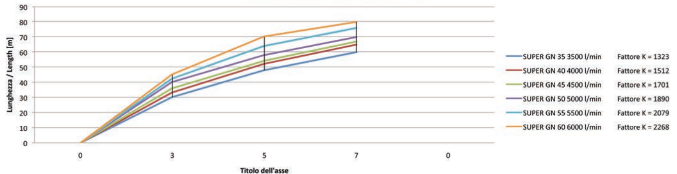
Grafico di gittata - Horizontal throw diagram Bocchello - Nozzle SUPER GN Gittate a getto pieno - Full jet horizontal throw Elevazione bocchello - Nozzle elevation 20° + 30°
