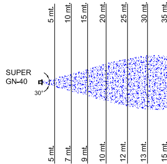
Grafico di gittata - Horizontal throw diagram Bocchello - Nozzle SUPER GN Gittate a getto nebulizzato - Fog jet horizontal throw Elevazione bocchello - Nozzle elevation 20° + 30°
