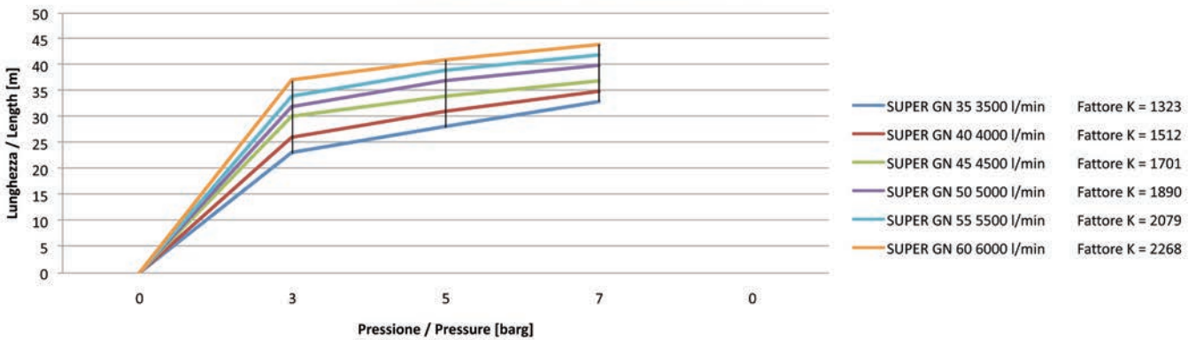
Grafico di gittata - Horizontal throw diagram Bocchello - Nozzle SUPER GN Gittate a getto nebulizzato - Fog jet horizontal throw Elevazione bocchello - Nozzle elevation 20° + 30°
