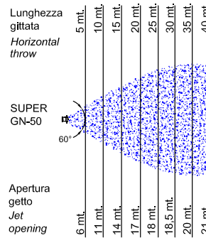
Grafico di gittata - Horizontal throw diagram Bocchello - Nozzle SUPER GN Gittate a getto nebulizzato - Fog jet horizontal throw Elevazione bocchello - Nozzle elevation 20° + 30°
